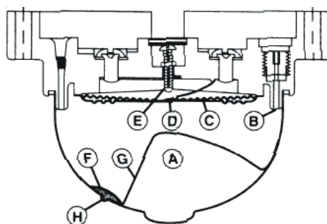
Slika 7.8 Termodiferencijalni javljač sa dijafragmom
