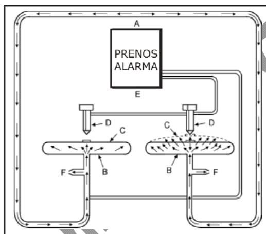
Slika 7.16 Linijski termodiferencijalni javljač
